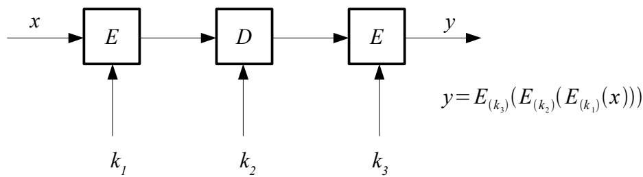
11. ábra: A 3DES EDE konfigurációban
