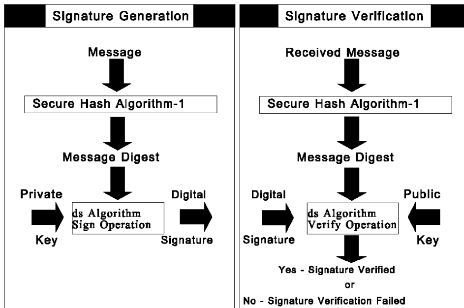
15. ábra: digitális aláírás készítése és ellenőrzése
