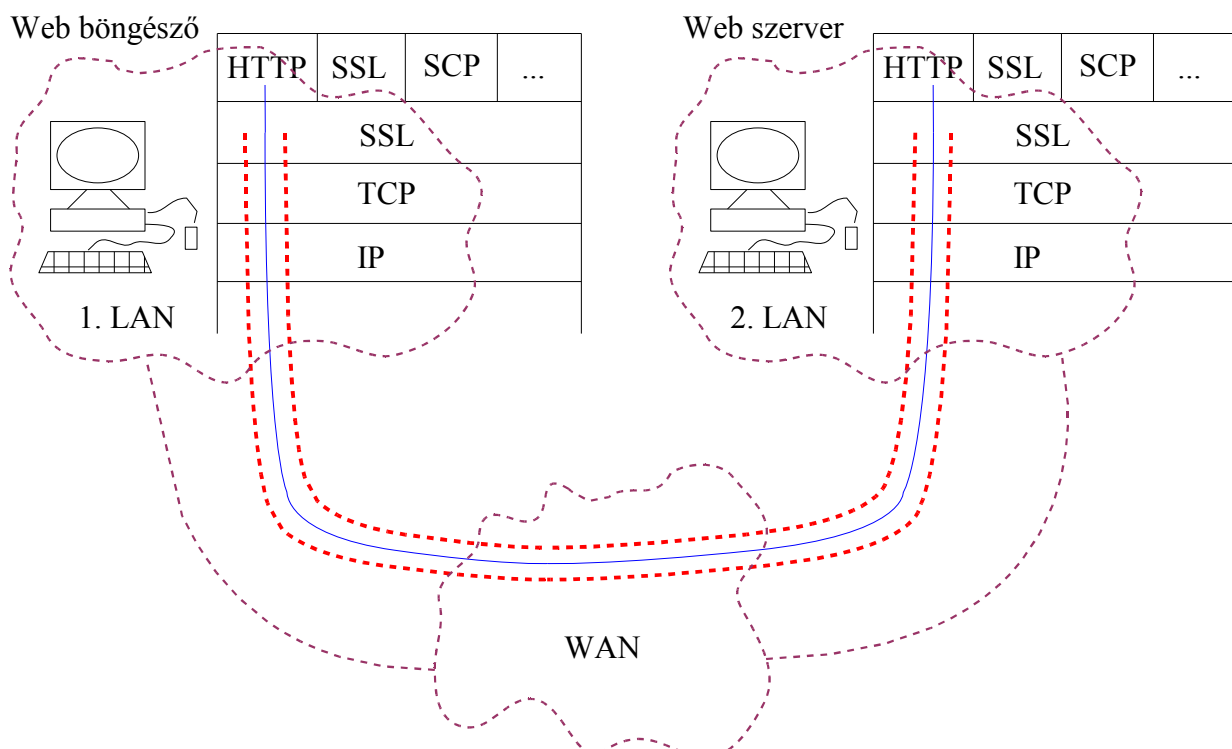
16. ábra: SSL kapcsolat
