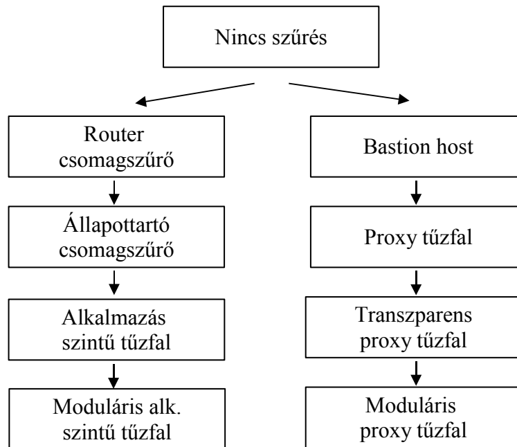
18. ábra: Tűzfalak fejlődése
