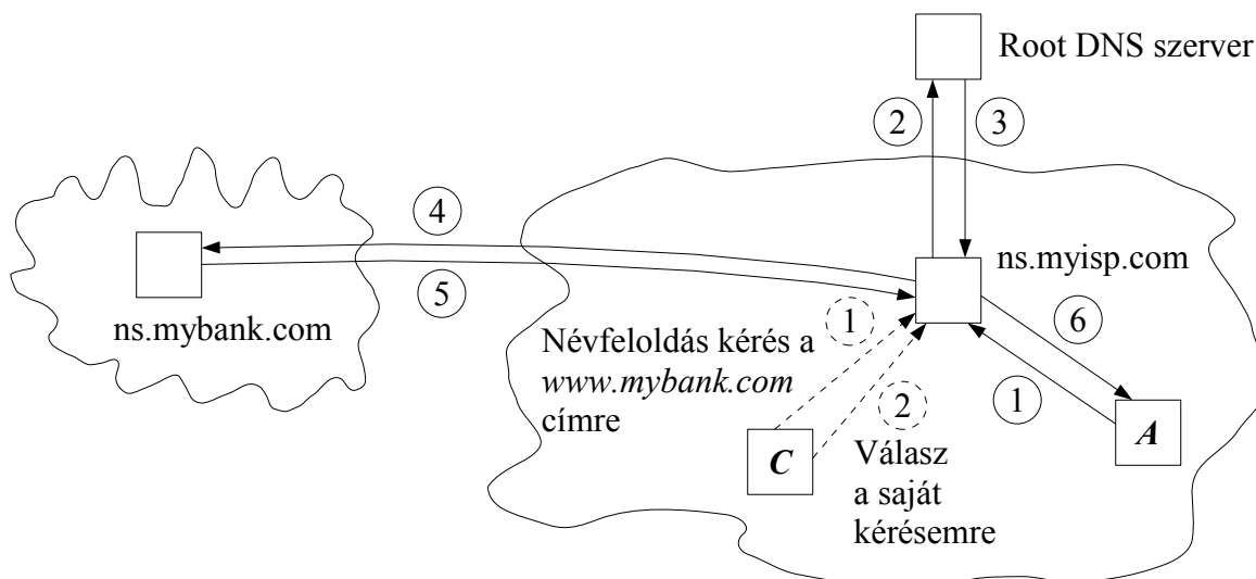
9. ábra: DNS (cache) elleni támadás
