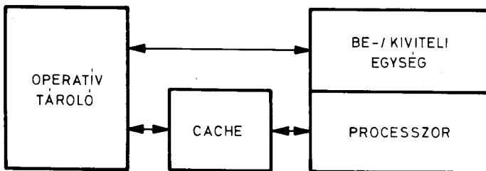
2.6. ábra. A cache helye a külvilág szempontjából: a) a cache az operatív tároló része, b) a cache a processzor része
