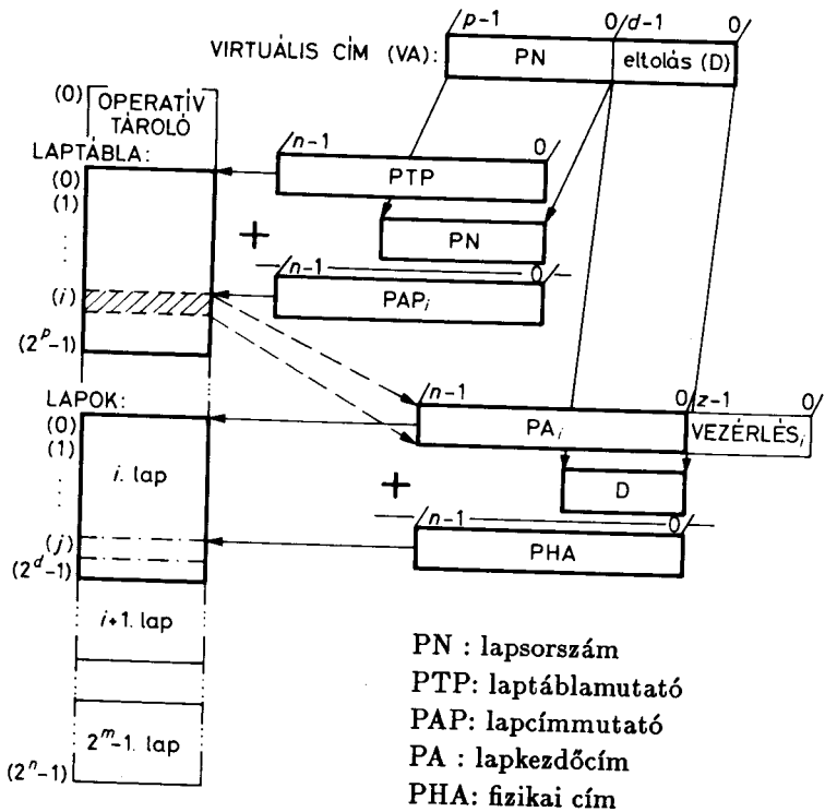
2.3. ábra. Címszámítás lapszervezésű virtuális tárolóban
