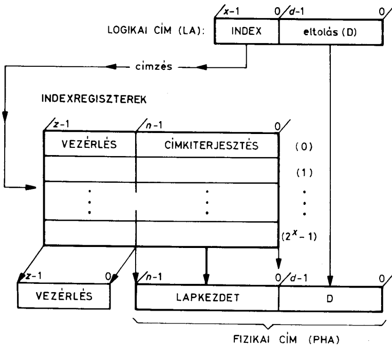
2.2. ábra. Az indexelt leképzés elve
