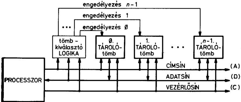
2.1. ábra. A tömbkapcsolás elve
