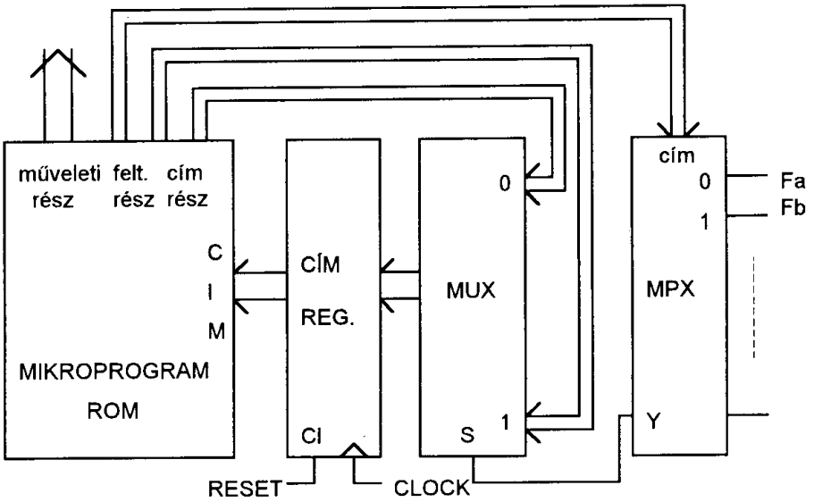
3.8. ábra. Két címrészből választó mikroprogramozott vezérlő
