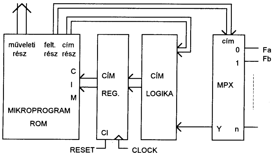
3.5. ábra. Mikroprogramozott vezérlő általános blokkműveletje
