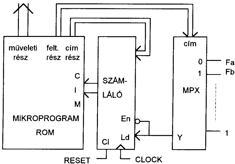
3.7. ábra. Számlálós címregiszterű mikroprogramozott vezérlő
