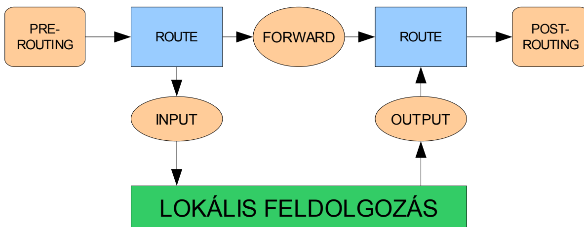
9. ábra: IP routing a 2.4.x kernelekben
