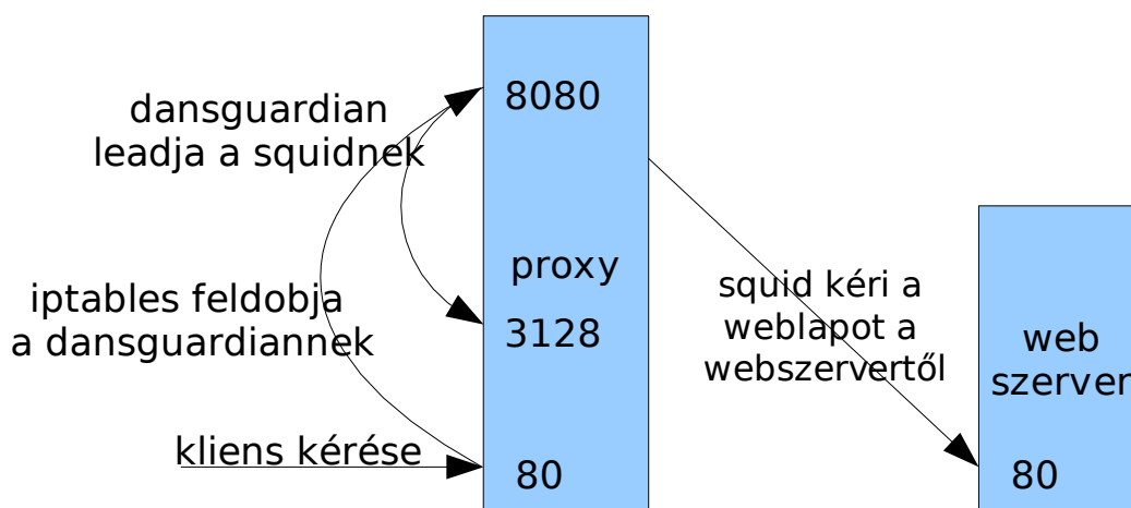
13. ábra: dansguardian squid működése
