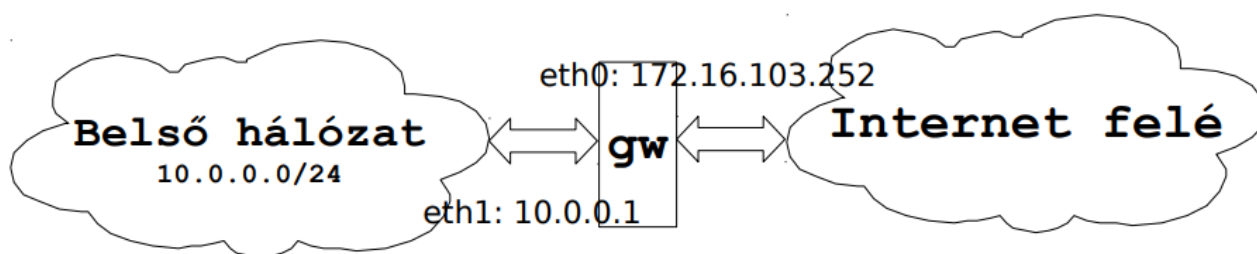
13. ábra: minta rendszer transparens proxy megvalósításához
