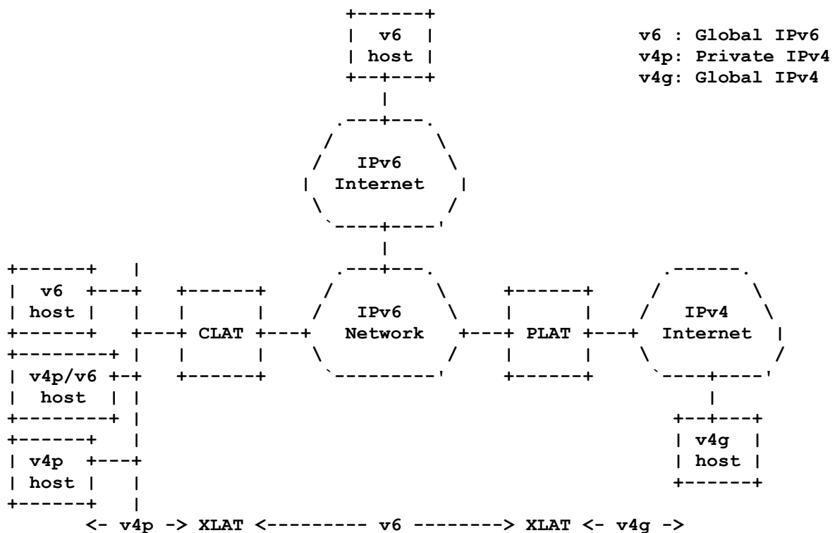
4. ábra: 464XLAT rendszer felépítése vezetékes hálózat esetén (RFC 6877)
