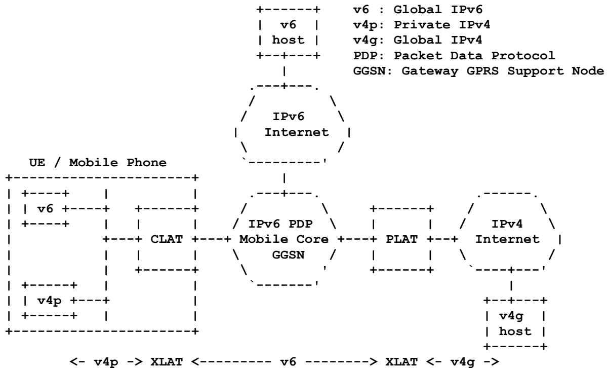
5. ábra: 464XLAT rendszer felépítése mobil hálózat esetén (RFC 6877)
